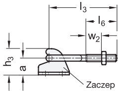
Typ TG z uchem mocującym
