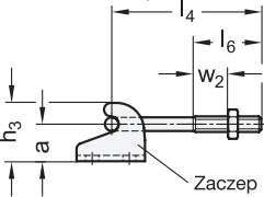
Typ TT z elementem mocującym w kształcie teowym
